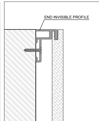
D END INVISIBLE PROFILE-INTERIOR
