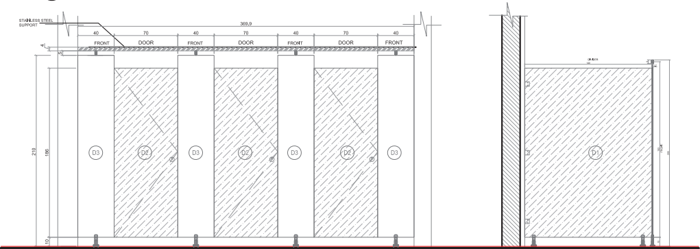
W.C - ELEVATION CUBICLES
